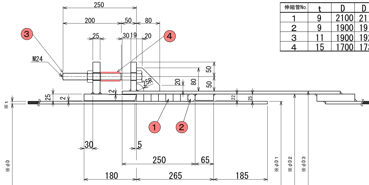
※寸法表
